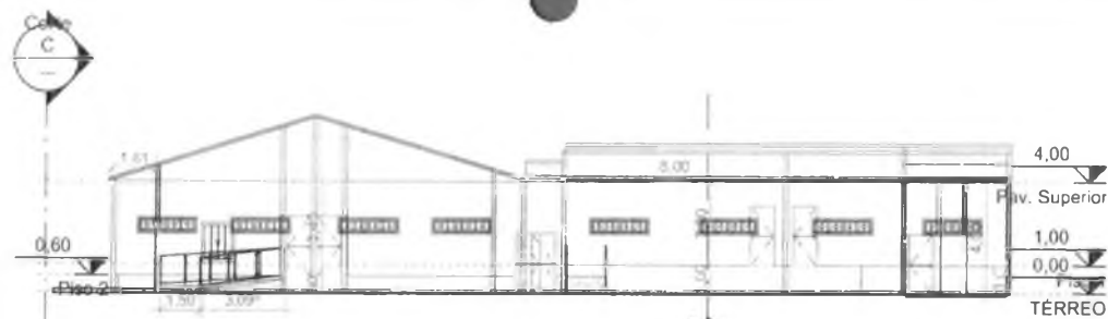
1 Corte A 1 : 200
